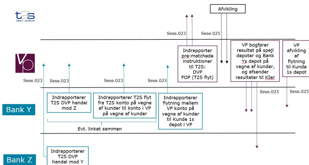
Figur 6 – Meddelelsesflow hvor Kunde 1 i bank Y køber fra bank Z
